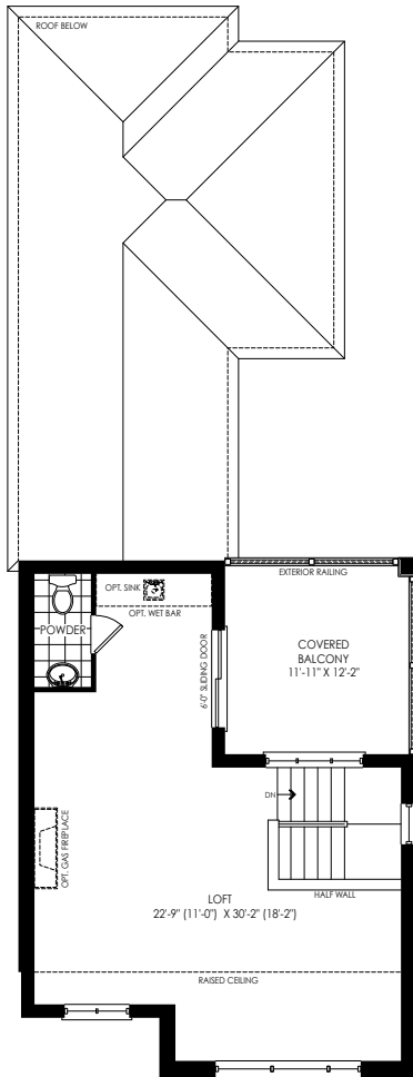
LOFT PLAN ELEV. 'A'
