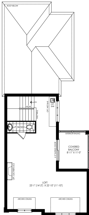
LOFT PLAN ELEV. 'D'
