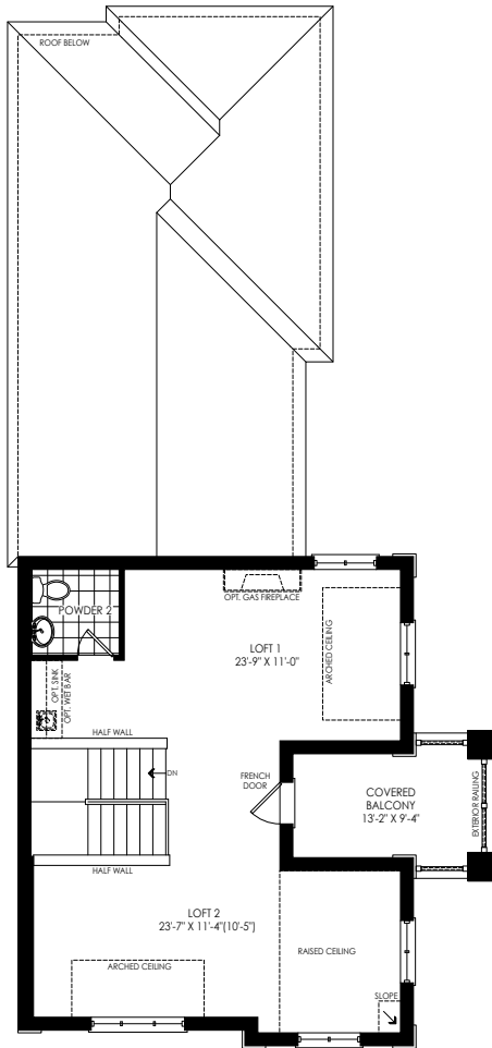
LOFT PLAN ELEV. 'D'
