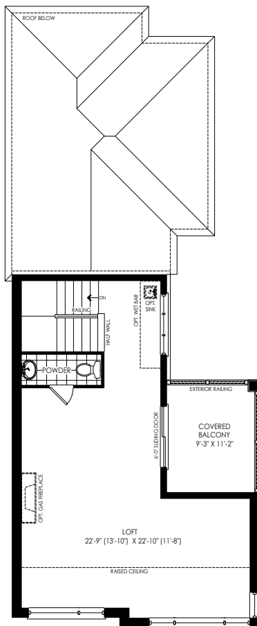
LOFT PLAN ELEV. 'A'
