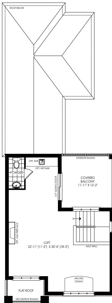
LOFT PLAN ELEV. 'D'
